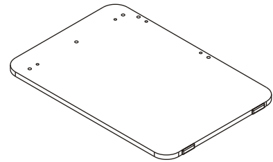
18.31.1201.018 x 1
